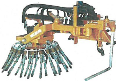
Gyomkefe
